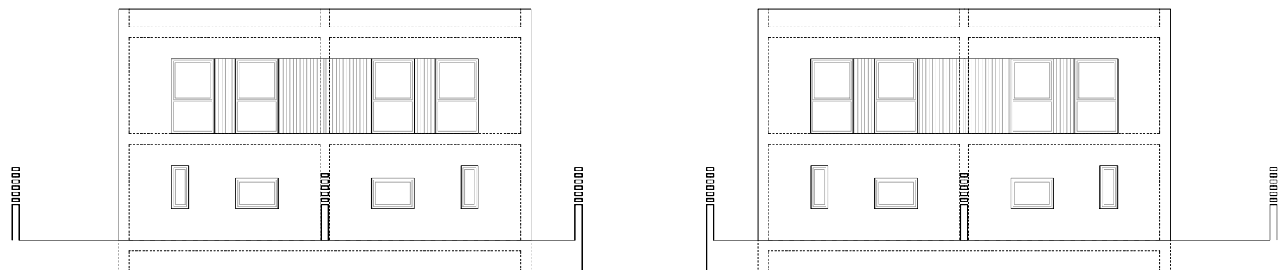
ALÇAT 2 - CARRER SANT JORDI - ALÇAT POSTERIOR
