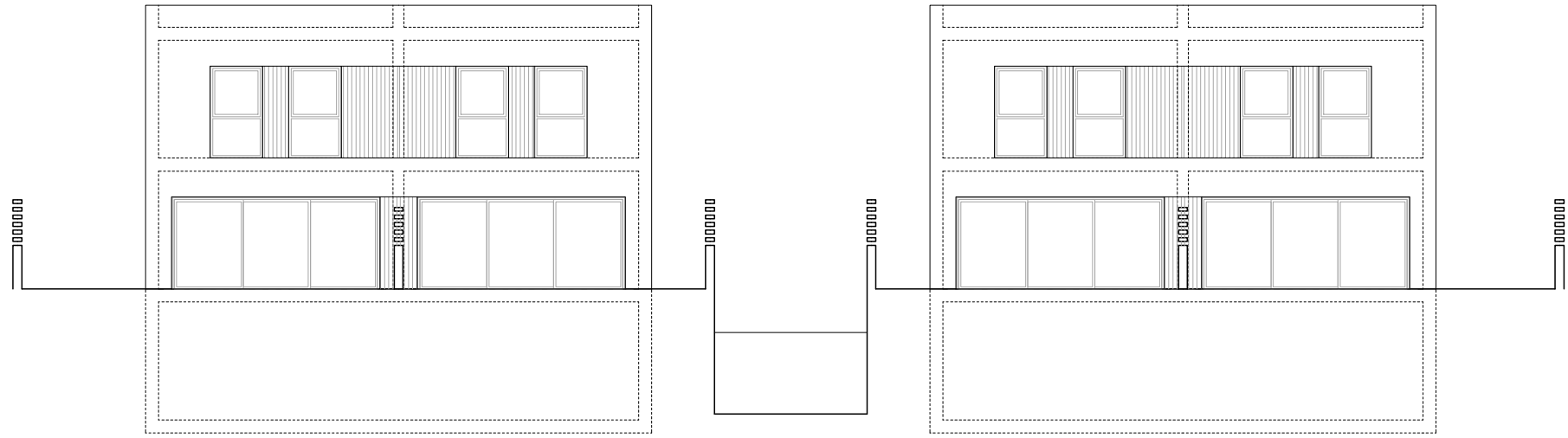
ALÇAT 3 - CARRER VERGE DE NÚRIA - ALÇAT POSTERIOR
