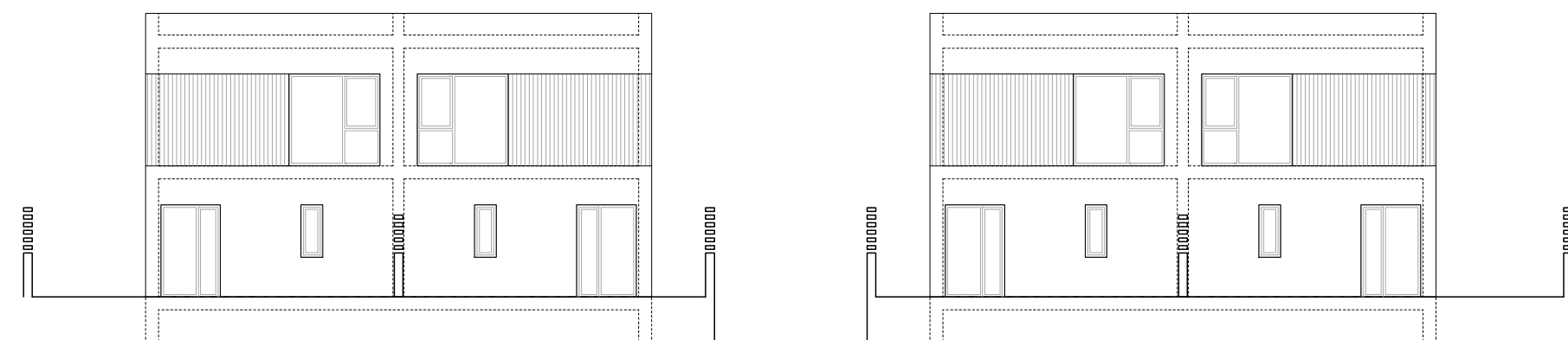
ALÇAT 4 - CARRER VERGE DE NÚRIA - ALÇAT FRONTAL
